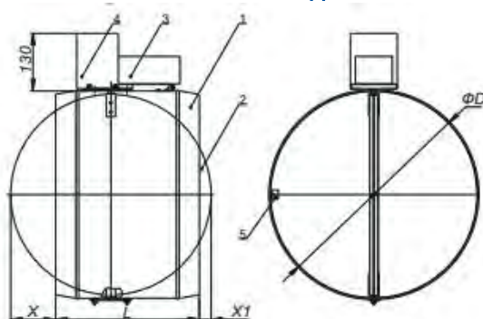
РКВ-1М/КПС-1М КАНАЛЬНЫЙ С ЭЛЕКТРОПРИВОДОМ
